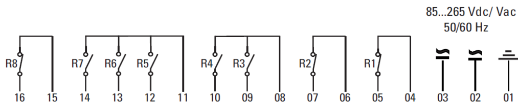
Figura 5 - Terminais entrada e saída do TM
