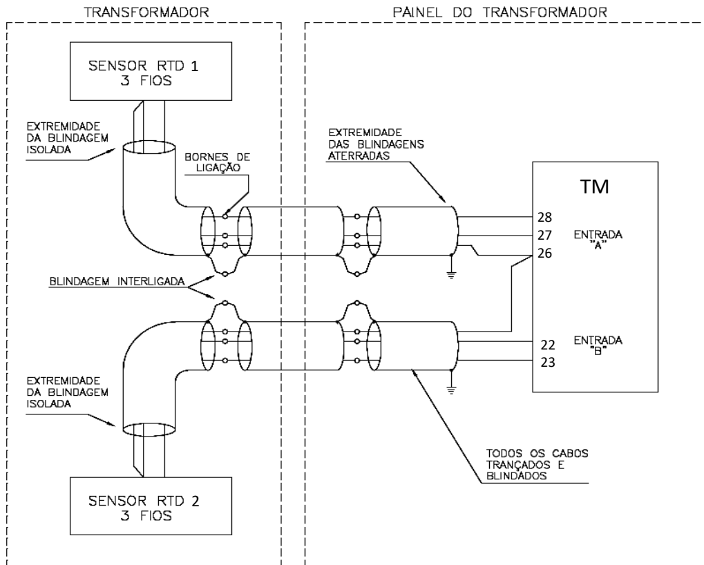
Figura 6 - Conexão da blindagem de interligação entre sensores RTD e TM
