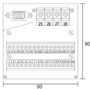
VISTA TRASEIRA
