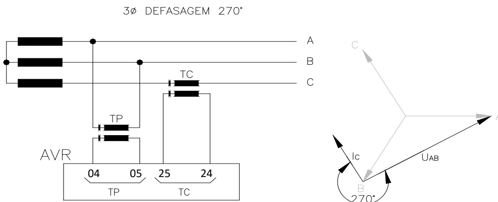
Figura 11 - Ligação de TP fase-fase, defasagem 270°
