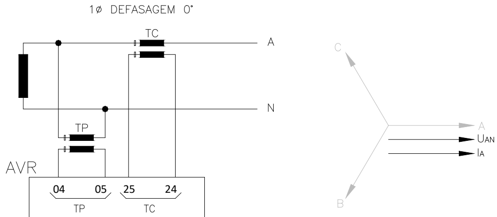
Figura 6 - Ligação para transformador monofásico, defasagem 0°
