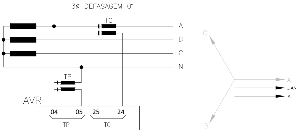
Figura 7 - Ligação de TP fase-neutro, defasagem 0°
