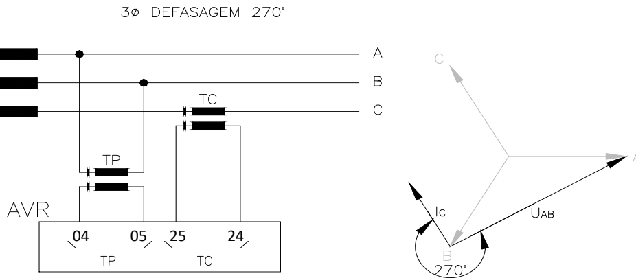
Figura 11 - Ligação de TP fase-fase, defasagem 270°
