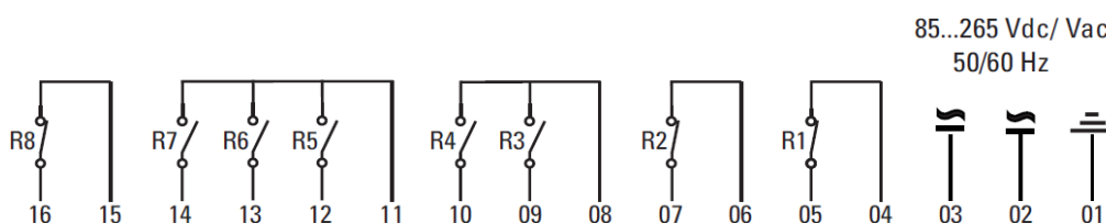
Figura 5 - Terminales de entrada y salida del TM
