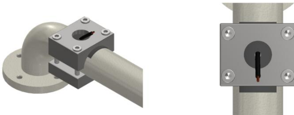
Figura 11 - Collar de derivación
