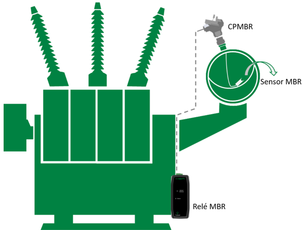
Figura 2 - Composición del sistema de detección de rotura de membrana/bolsa
