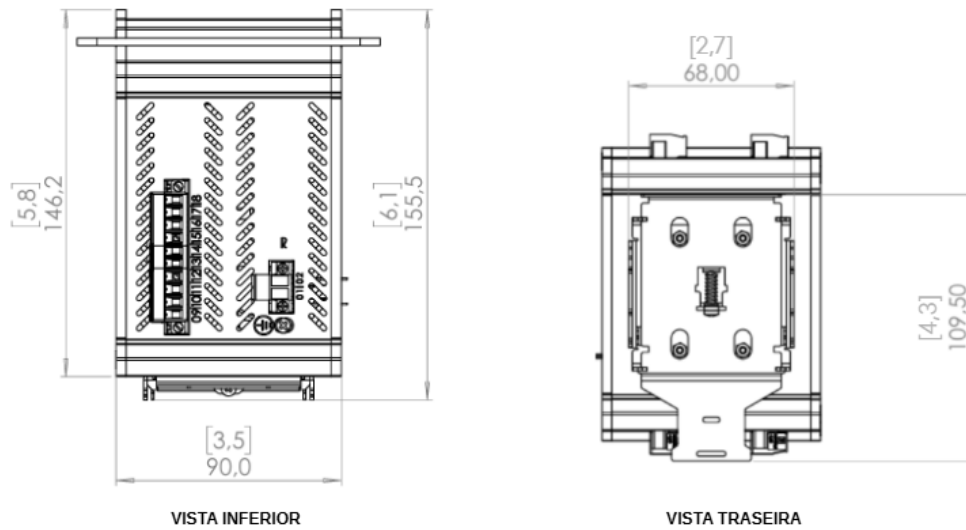
Figura 3 - Vista inferior e traseira
