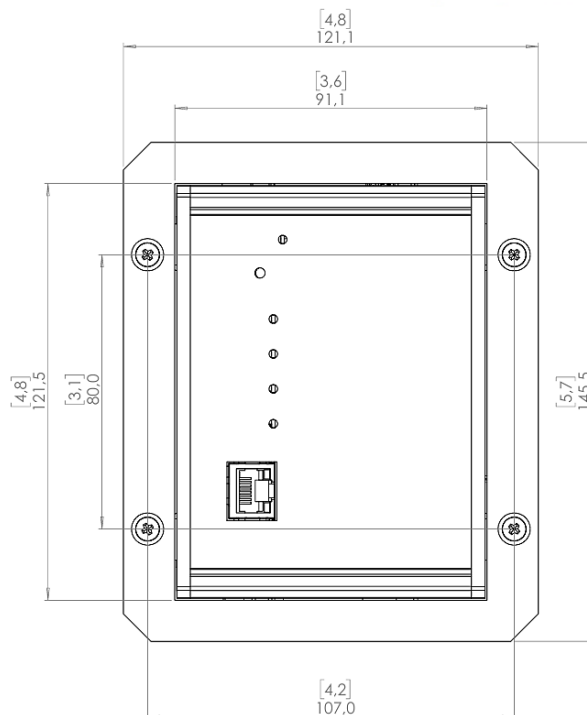
Figura 5 - Moldura para instalação em painel
