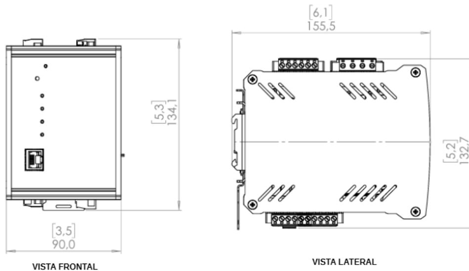
Figura 4 - Vista frontal e lateral
