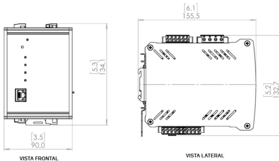
Figura 8 - Vista frontal e lateral
