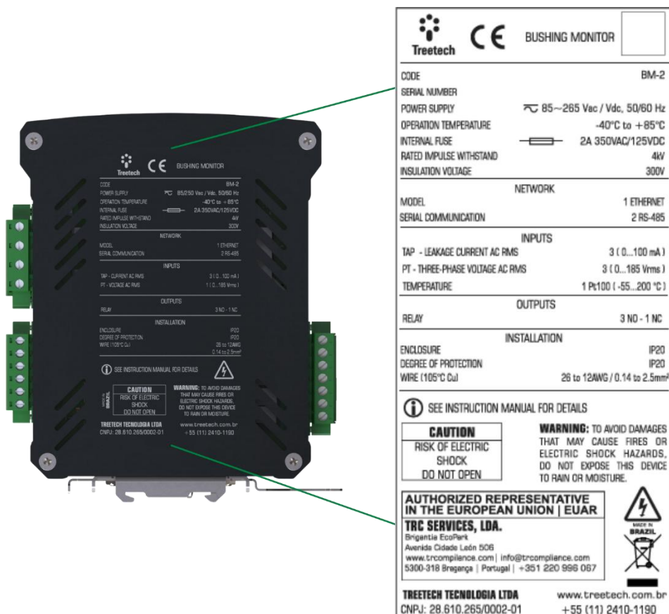
Figura 11 - Etiqueta com marcação CE
