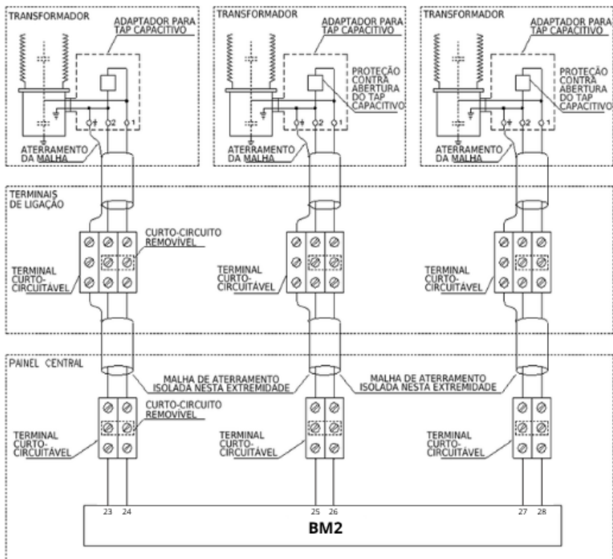
Figura 15 - Detalhes de conexão e aterramento
