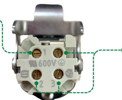
Figura 16 - Borne da tomada do adaptador de TAP
