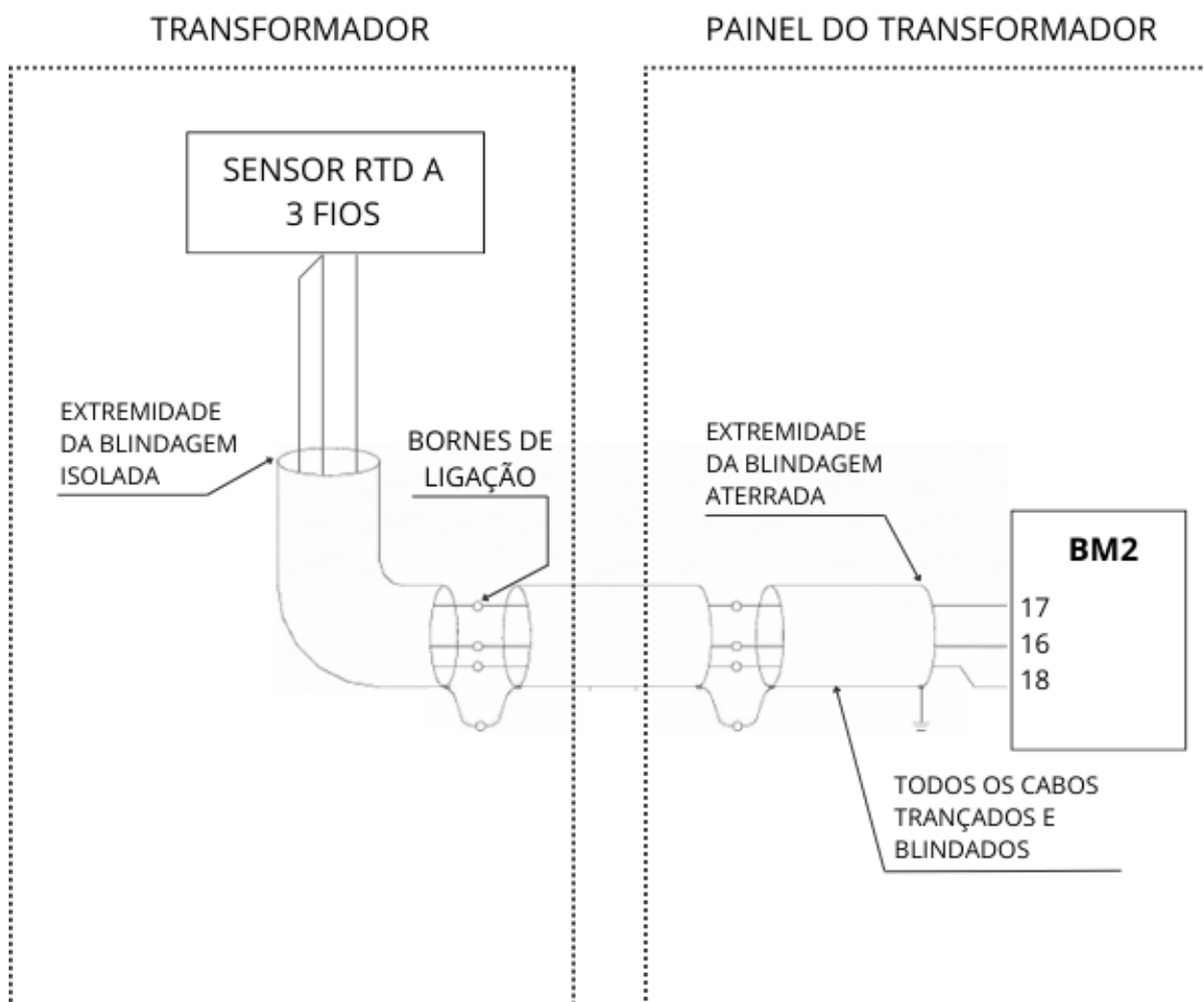
Figura 13 - Detalhes de conexão e aterramento dos cabos e blindagem
