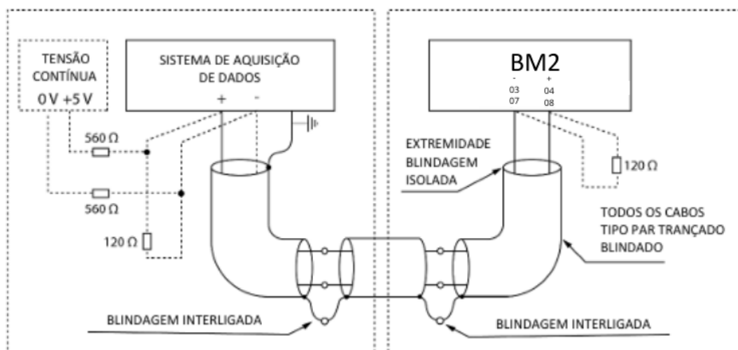
Figura 12 - Conexão e aterramento da blindagem da comunicação serial RS-485
