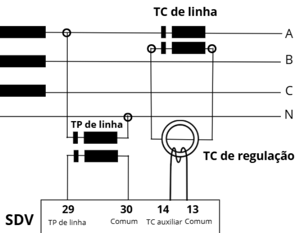
Figura 15 – Ligação de TP fase-neutro, defasagem 0°
