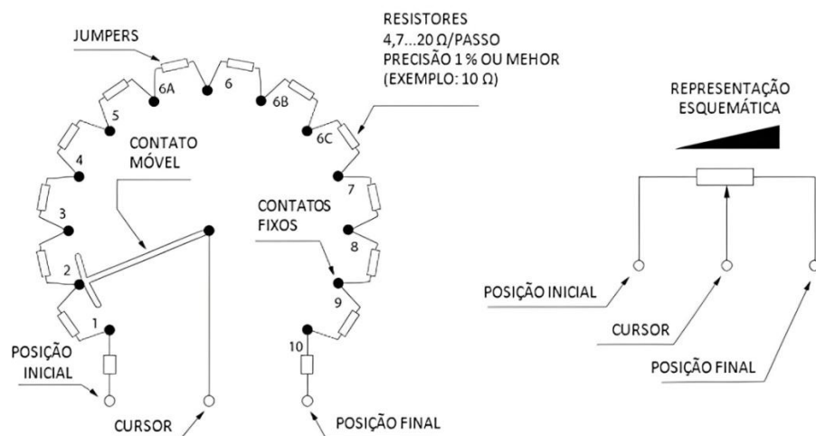
Figura 22 – Configuração dos resistores do transmissor potenciométrico nas posições intermediárias do CDC
