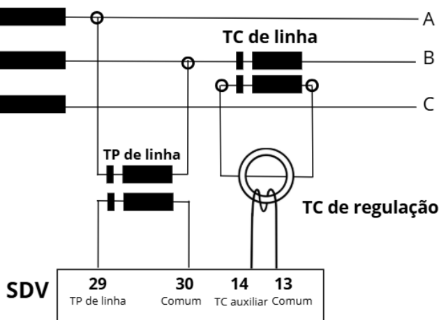
Figura 17 – Ligação de TP fase-fase, defasagem 150°
