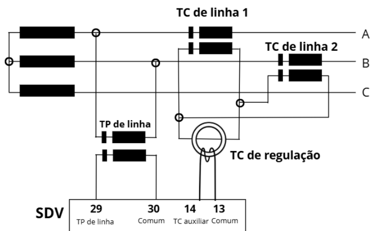
Figura 16 – Ligação de TP fase-fase, defasagem 0°
