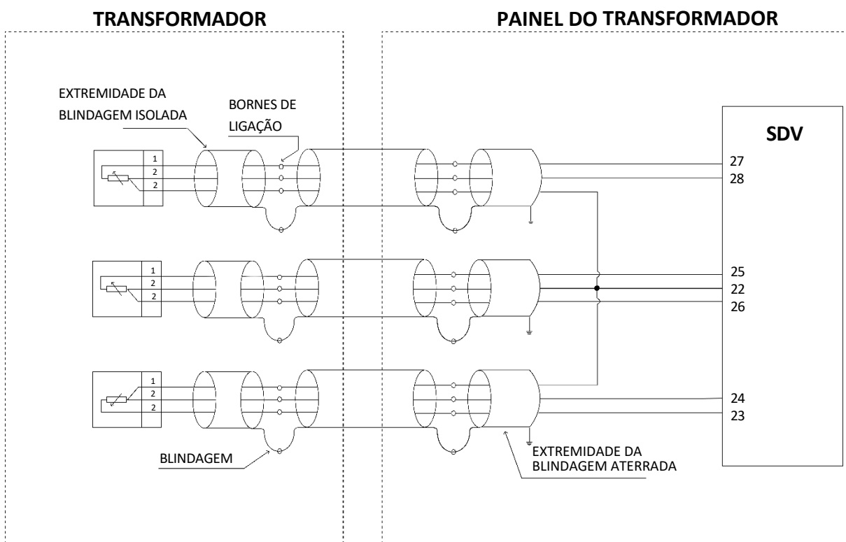
Figura 20 – Conexão da blindagem da interligação entre sensores RTD e o SDV
