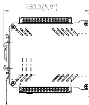
VISTA LATERAL
